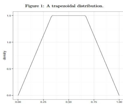
Fig 1:Trapizoidal function
